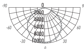
PSL 08 100w 120°
